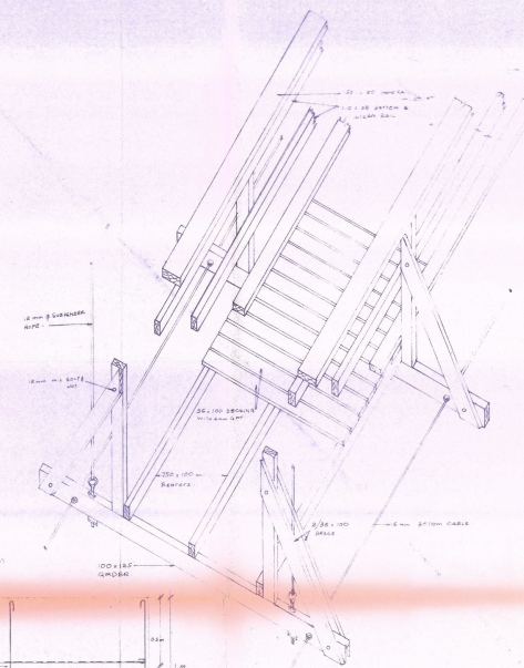
ISOMETRIK VIEW SCALE: 1:20
